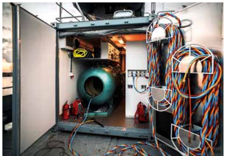
Контейнеризированная водолазная станция
